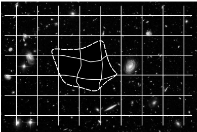
a / Einstein’s hole argument.
